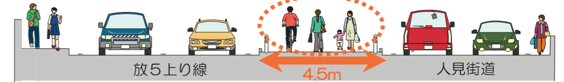
図 新たな橋の整備前後の横断面イメージ
