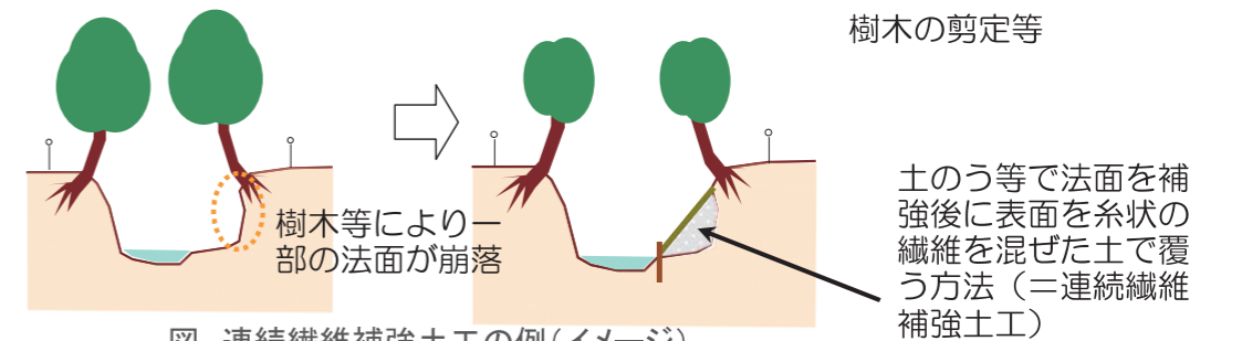
図 連続繊維補強土工の例(イメージ)
