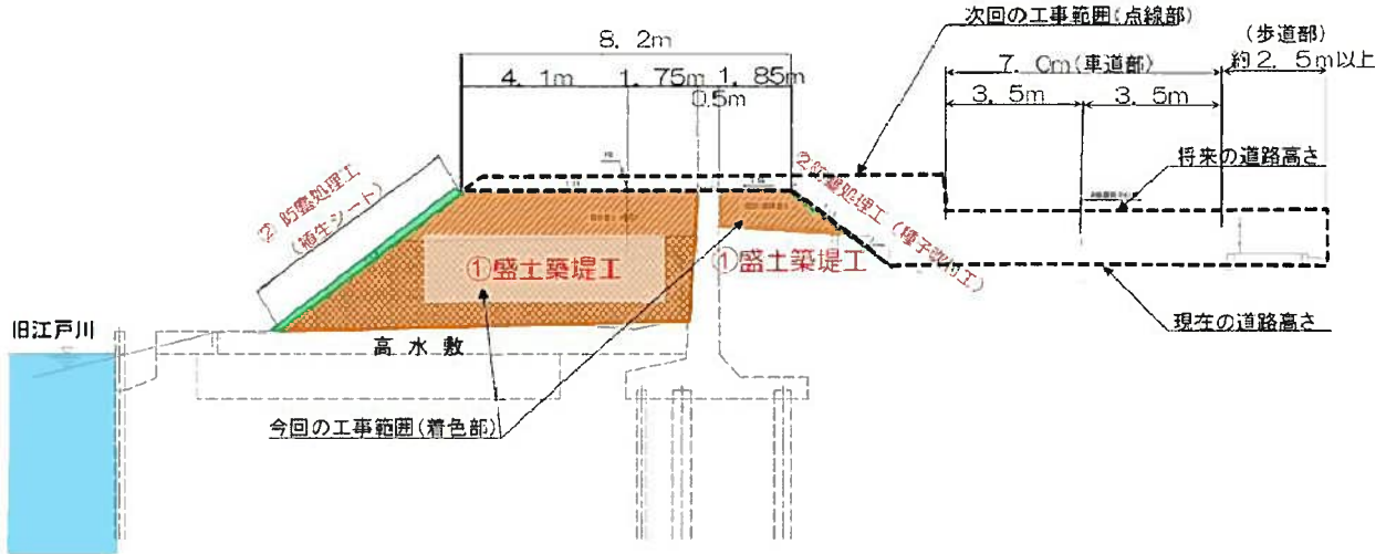
施工断面図
