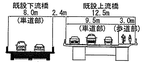
断面図 (既設橋)
