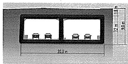
トンネル断面図
