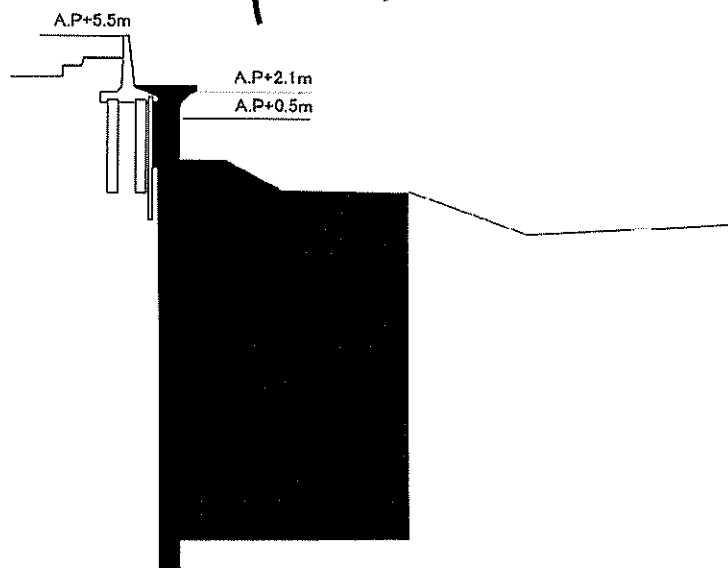
標準断面図
