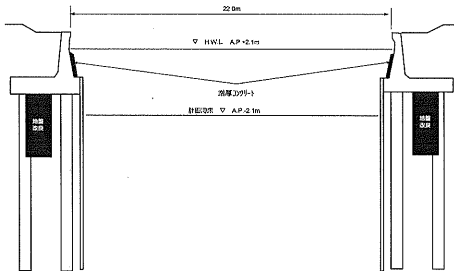
標準断面図
