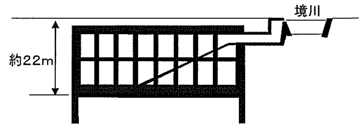
標準断面図
