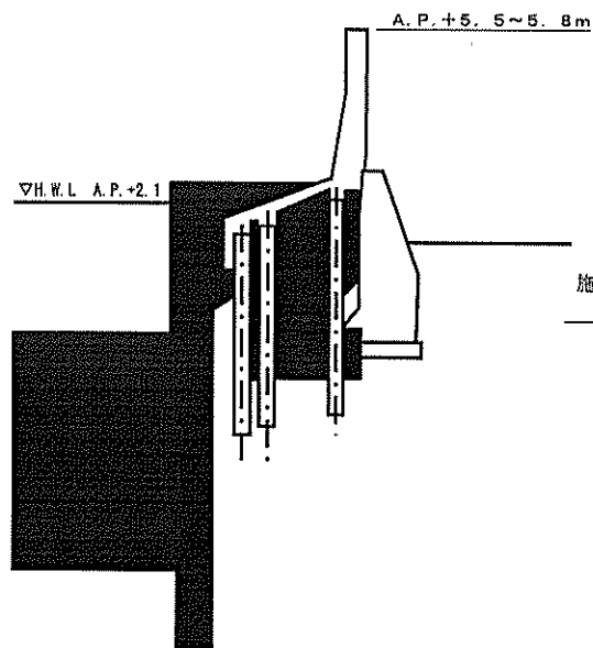
標準断面図
