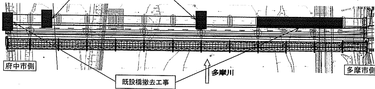
平面図
