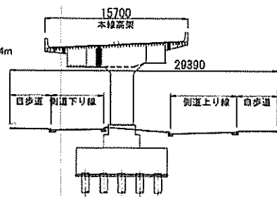
勝どき高架橋断面図
