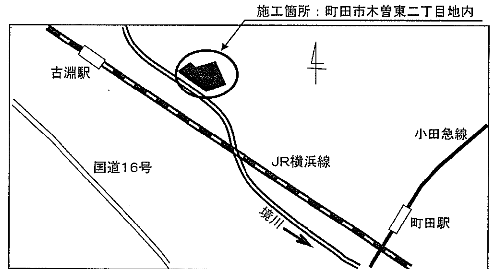
案内図
