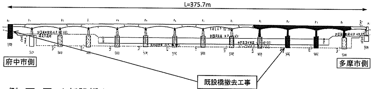
側面図 (新設橋)
