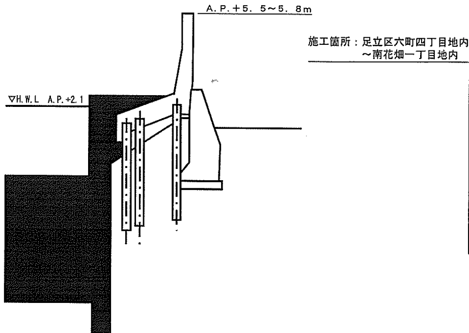
標準断面図
