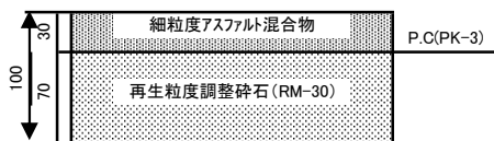
歩道舗装 10型 (非透水)
