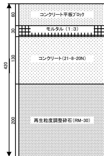
コンクリート平板乗入れ舗装 (D)
