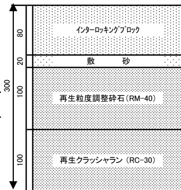
インターロッキングブロック乗入れ舗装 (A,B,C)
