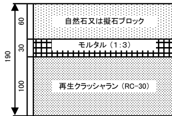
自然石(擬石ブロック)舗装
