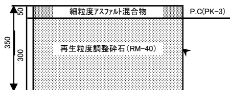
乗入れ舗装 アスコン35型 (A,B,C)
