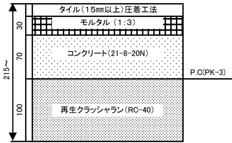
タイル舗装(一般部)
