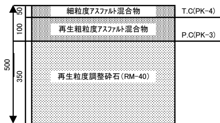
乗入れ舗装 アスコン50型 (D)
