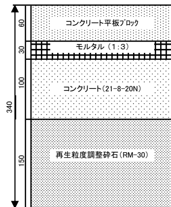
コンクリート平板乗入れ舗装 (A,B,C)
