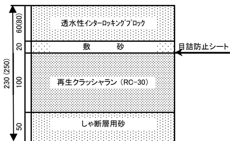
インターロッキング舗装(透水性)
