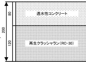
透水性コンクリート舗装
