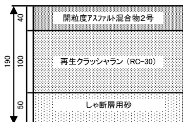
歩道舗装 19型 (透水性)
