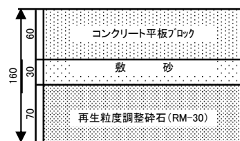
コンクリート平板舗装(非透水)
