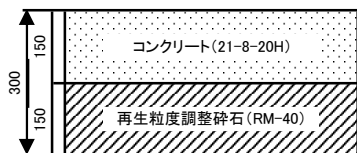
乗入れ舗装 セムコン30型 (A,B,C)
