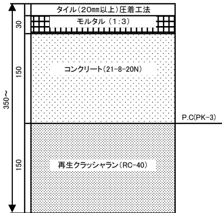
タイル乗入れ舗装 (A,B,C)
