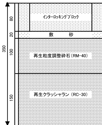
インターロッキングブロック乗入れ舗装 (D)
