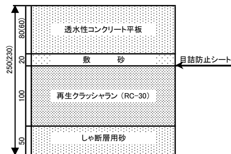
コンクリート平板舗装(透水性)
