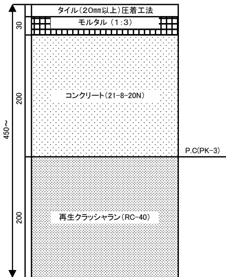
タイル乗入れ舗装 (D)
