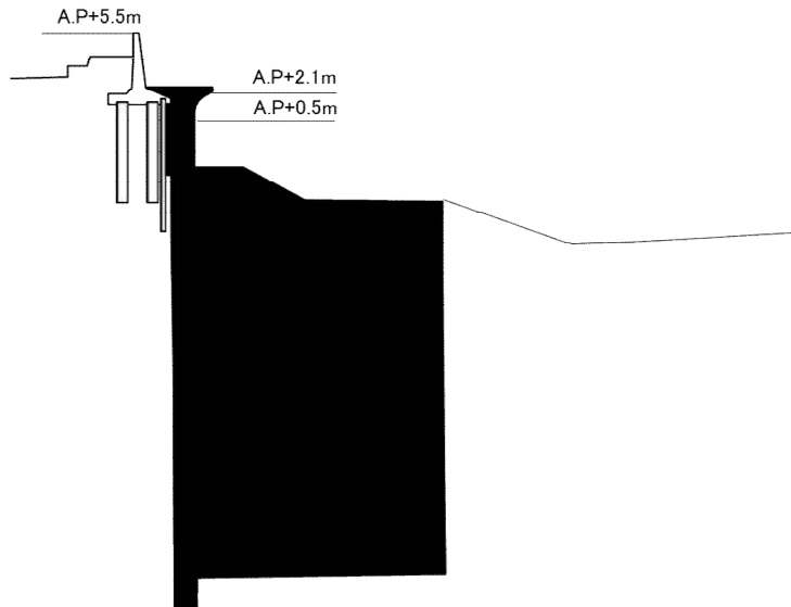
標準断面図
