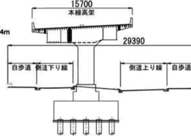
勝どき高架橋断面図
