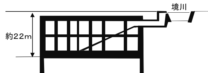
標準断面図
