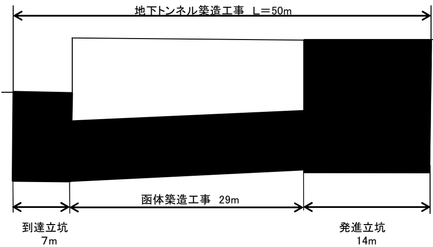
側面図
