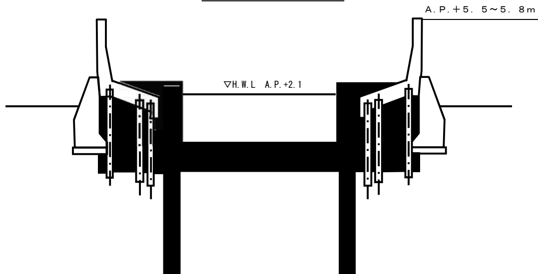
標準断面図
