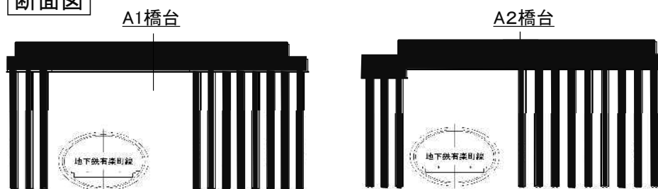
断面図
