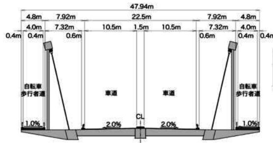
築地大橋断面図
