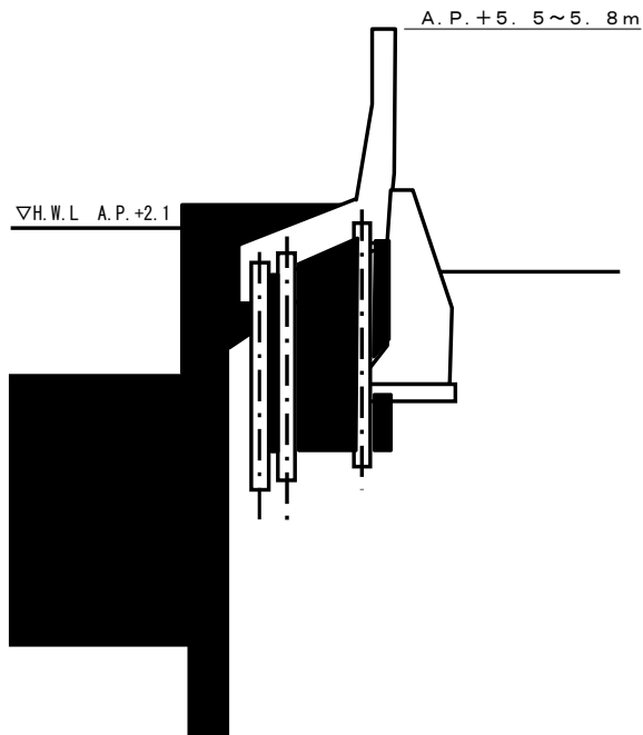
標準断面図
