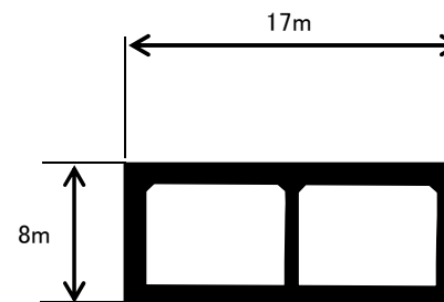
横断面図
