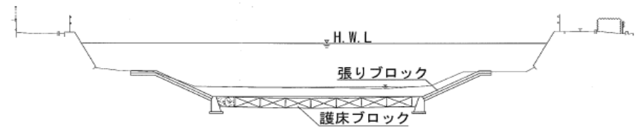
A-A' 断面図
