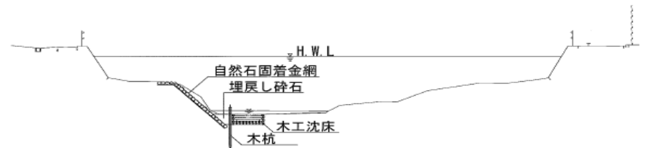
B-B' 断面図
