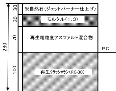
自然石舗装(一般部)
