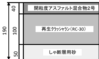
歩道舗装 19型 (透水性)
