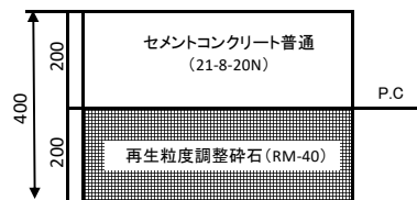
乗入れ舗装 セモン40型 (D型)
