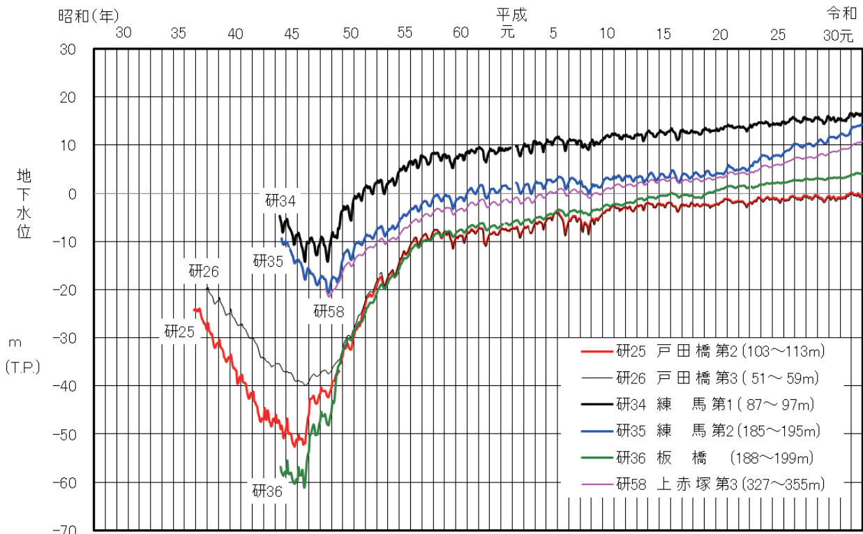
図-9 主な観測井の地下水位変動図（板橋区、練馬区）
