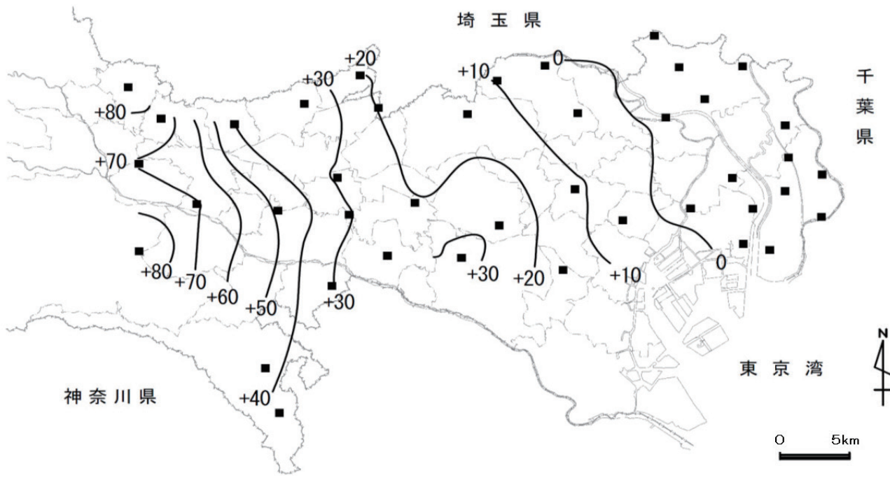
図-4 令和2年末の地下水位等高線図
