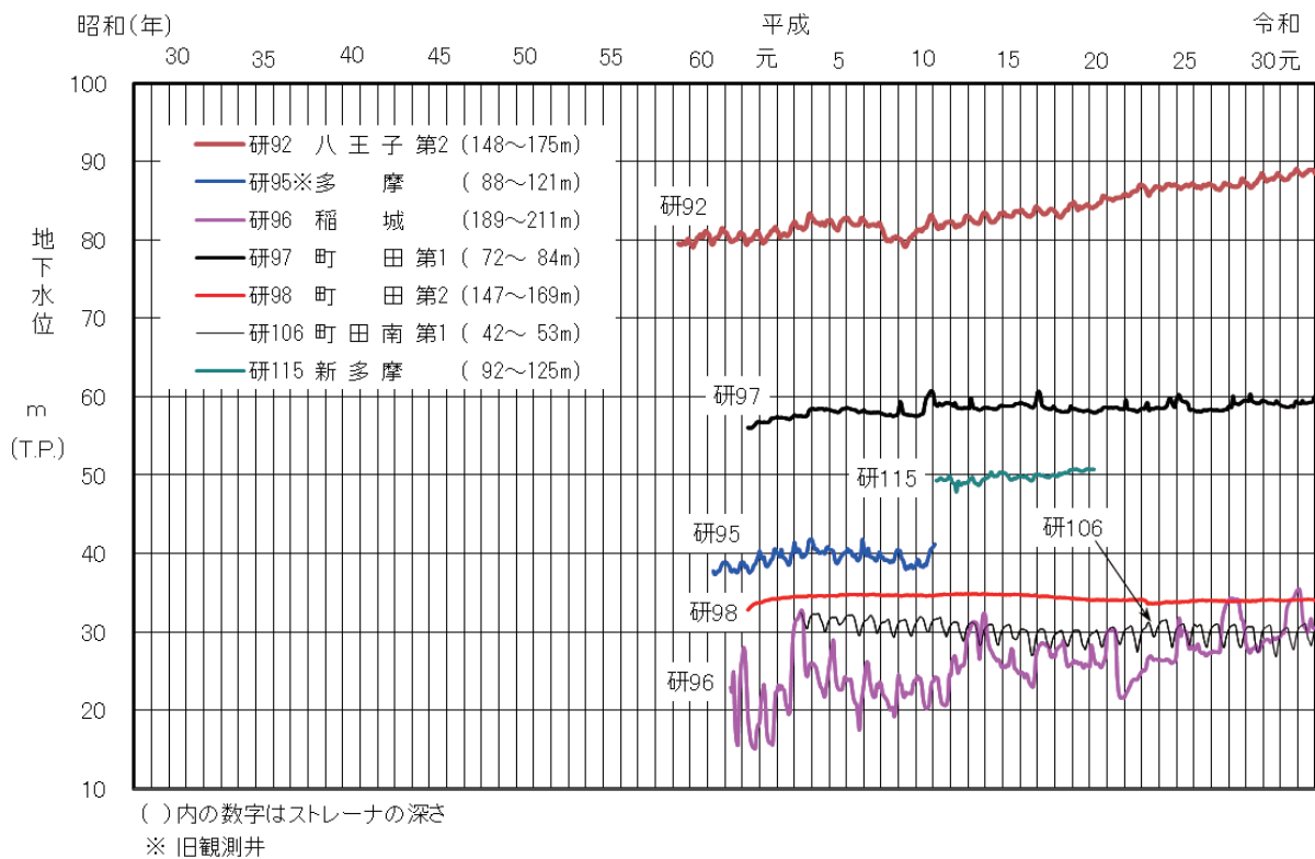
図-13 主な観測井の地下水水位変動図（八王子市、多摩市、稲城市、町田市）
