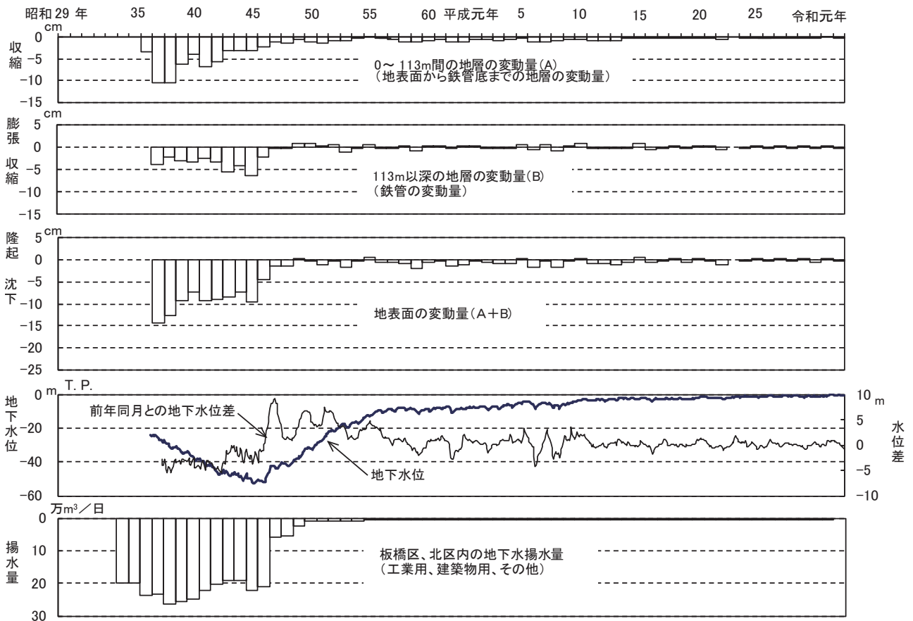
図-18 戸田橋第2観測井（113m井）における地盤変動量と地下水位との関係
