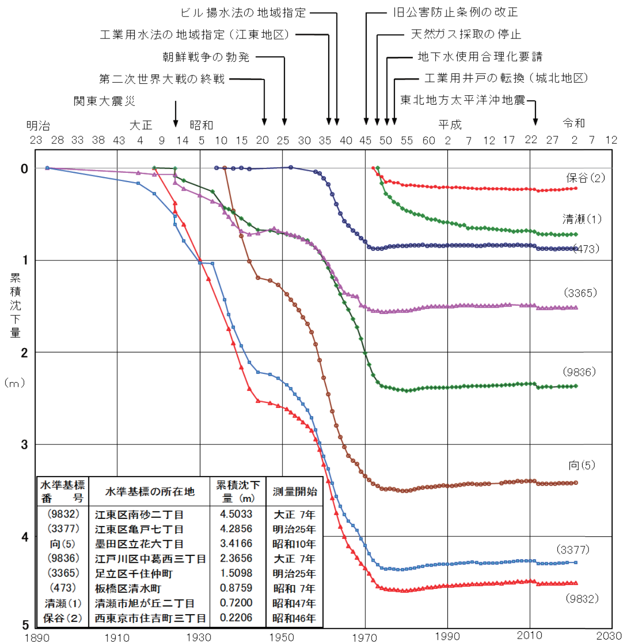
図-15 主要水準基標の累積沈下量図
