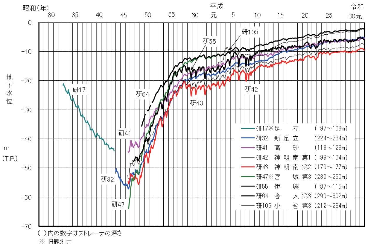
図-8 主な観測井の地下水水位変動図（足立区、葛飾区）
