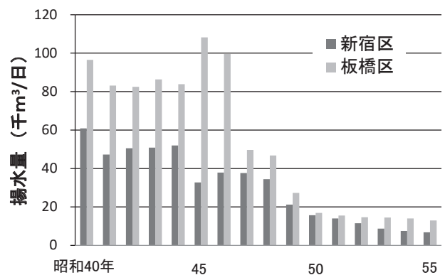
図-14 新宿区と板橋区での地下水揚水量の推移 注) 昭和45年までは地下水揚水量実態調査 2) 、46年以降は都内の地下水揚水の実態 3) による。
