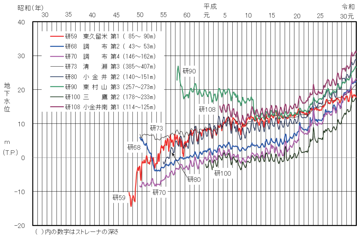
図-11 主な観測井の地下水水位変動図（東久留米市、清瀬市、東村山市、小金井市、調布市、三鷹市）
