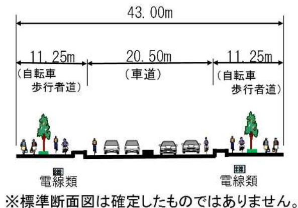
標準断面図
