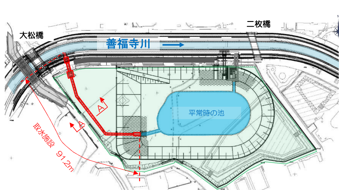
全体平面図
