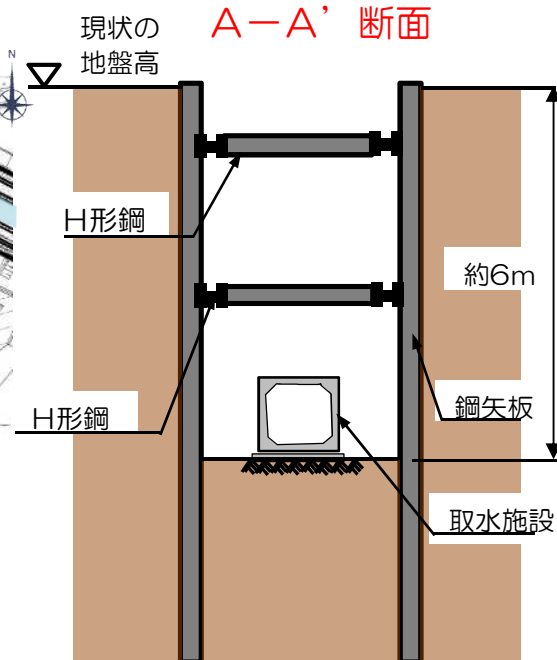
断面図
