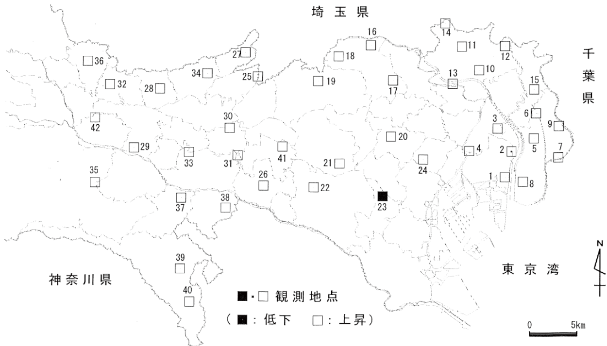
図-6 令和3年の地下水位変動状況図
