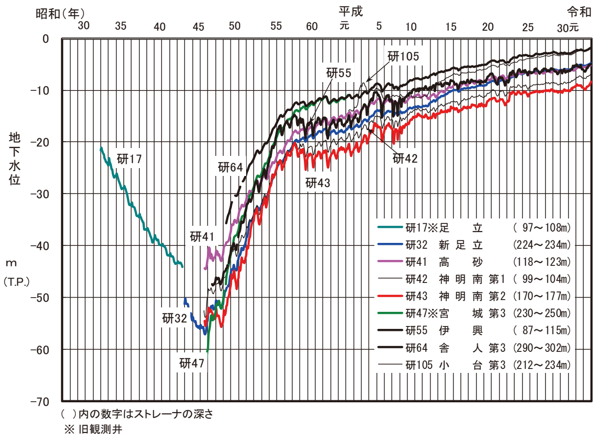
図-9 主な観測井の地下水位変動図（足立区、葛飾区）
