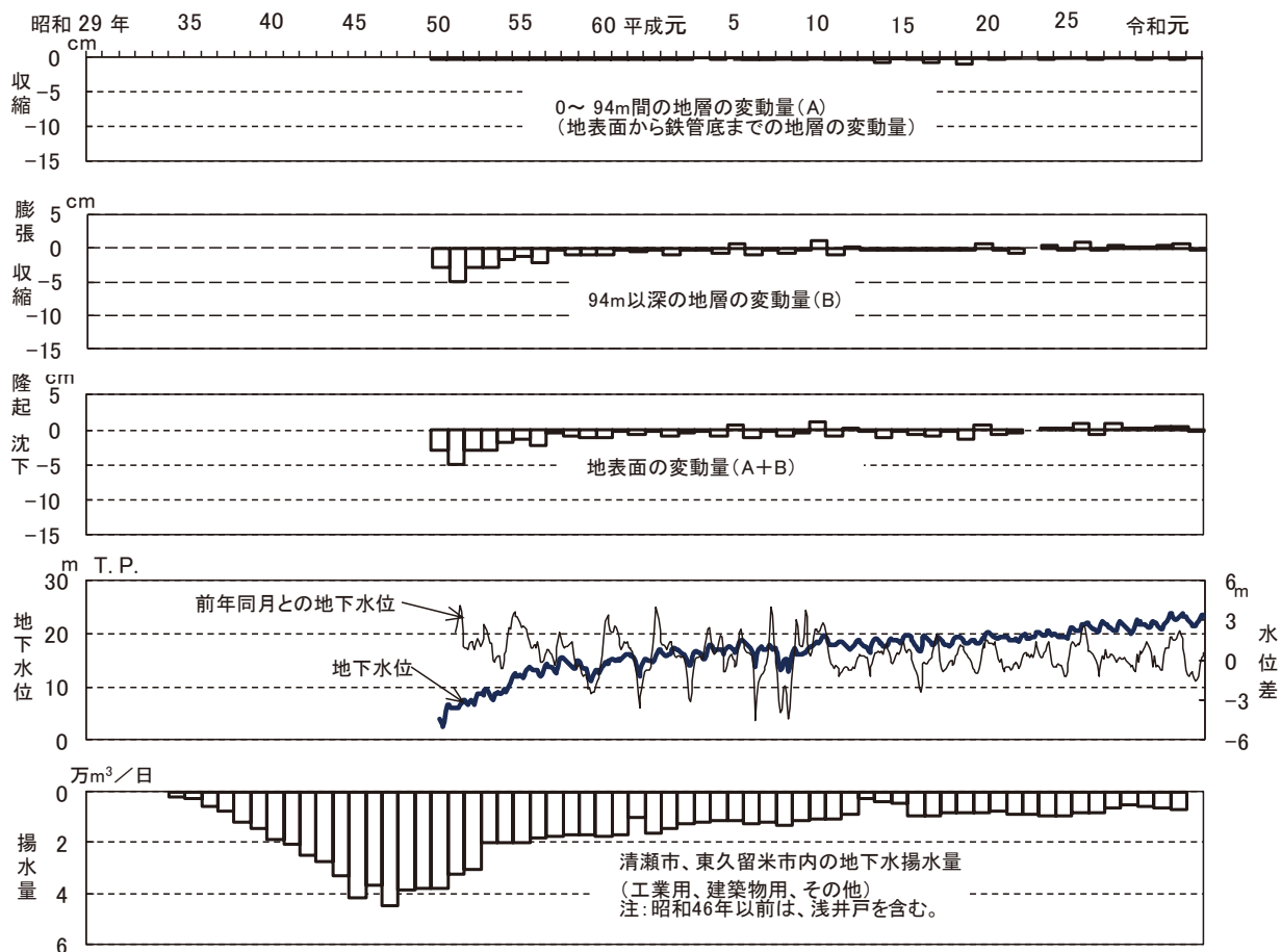
図-20 清瀬第1観測井（94m井）における地盤変動量と地下水位との関係
