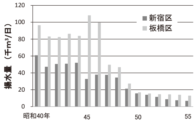
図-15 新宿区と板橋区での地下水揚水量の推移 注) 昭和45年までは地下水揚水量実態調査 2) 、46年以降は都内の地下水揚水の実態 3) による。
