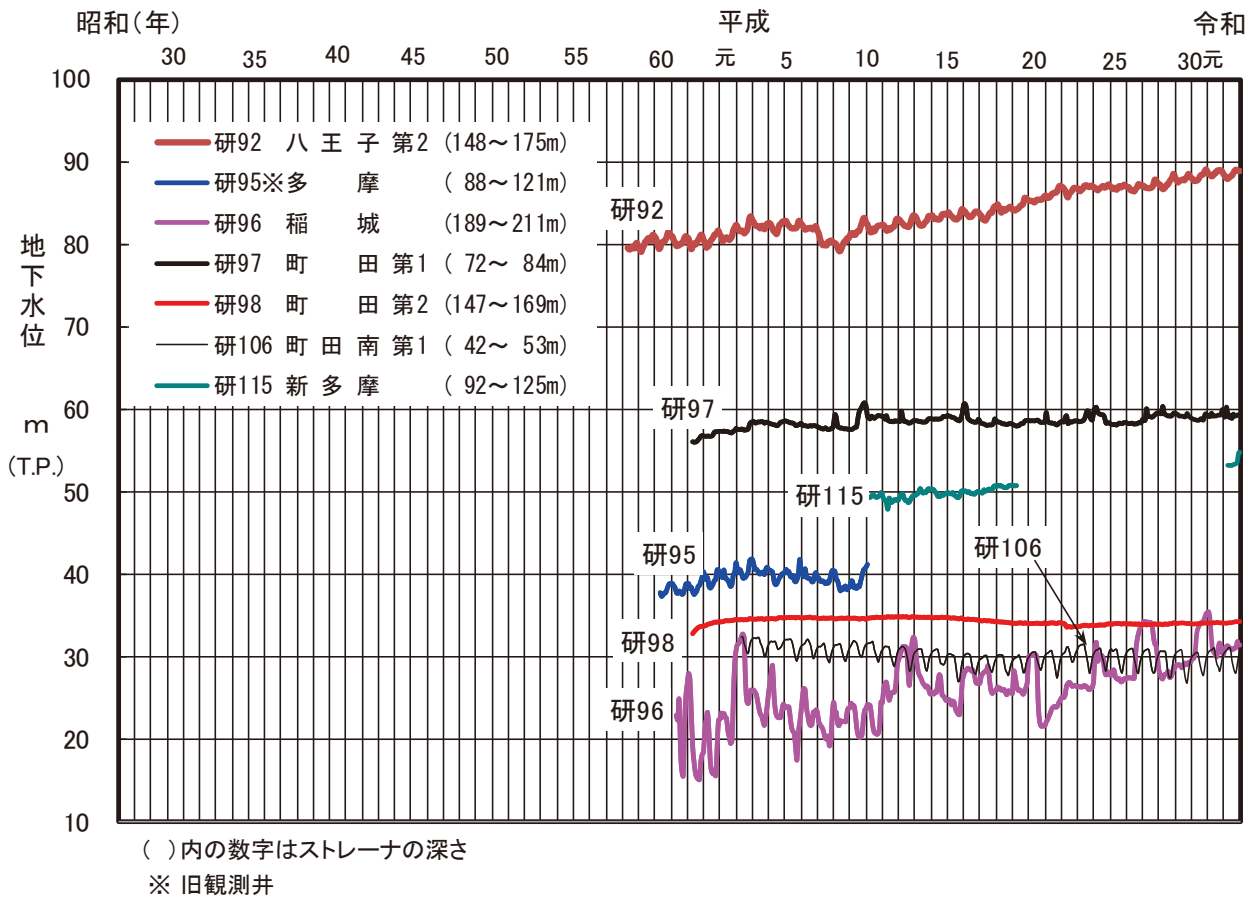
図-14 主な観測井の地下水位変動図（八王子市、多摩市、稲城市、町田市）
