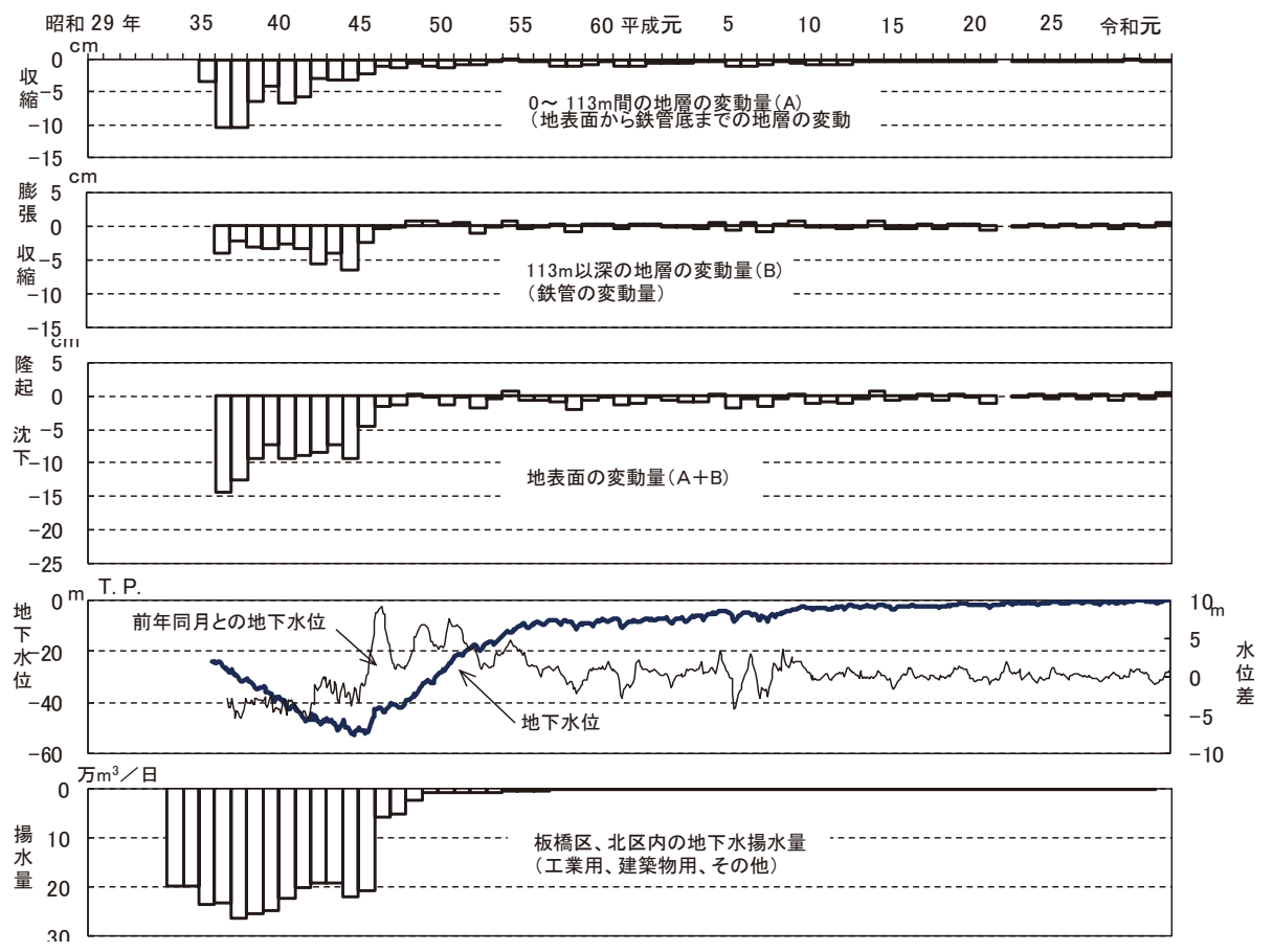
図-19 戸田橋第2観測井(113m井)における地盤変動量と地下水位との関係
