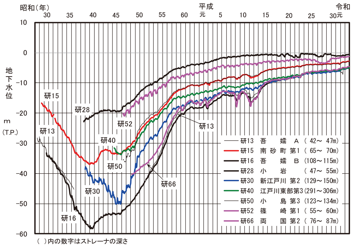
図-8 主な観測井の地下水位変動図（江東区、墨田区、江戸川区）
