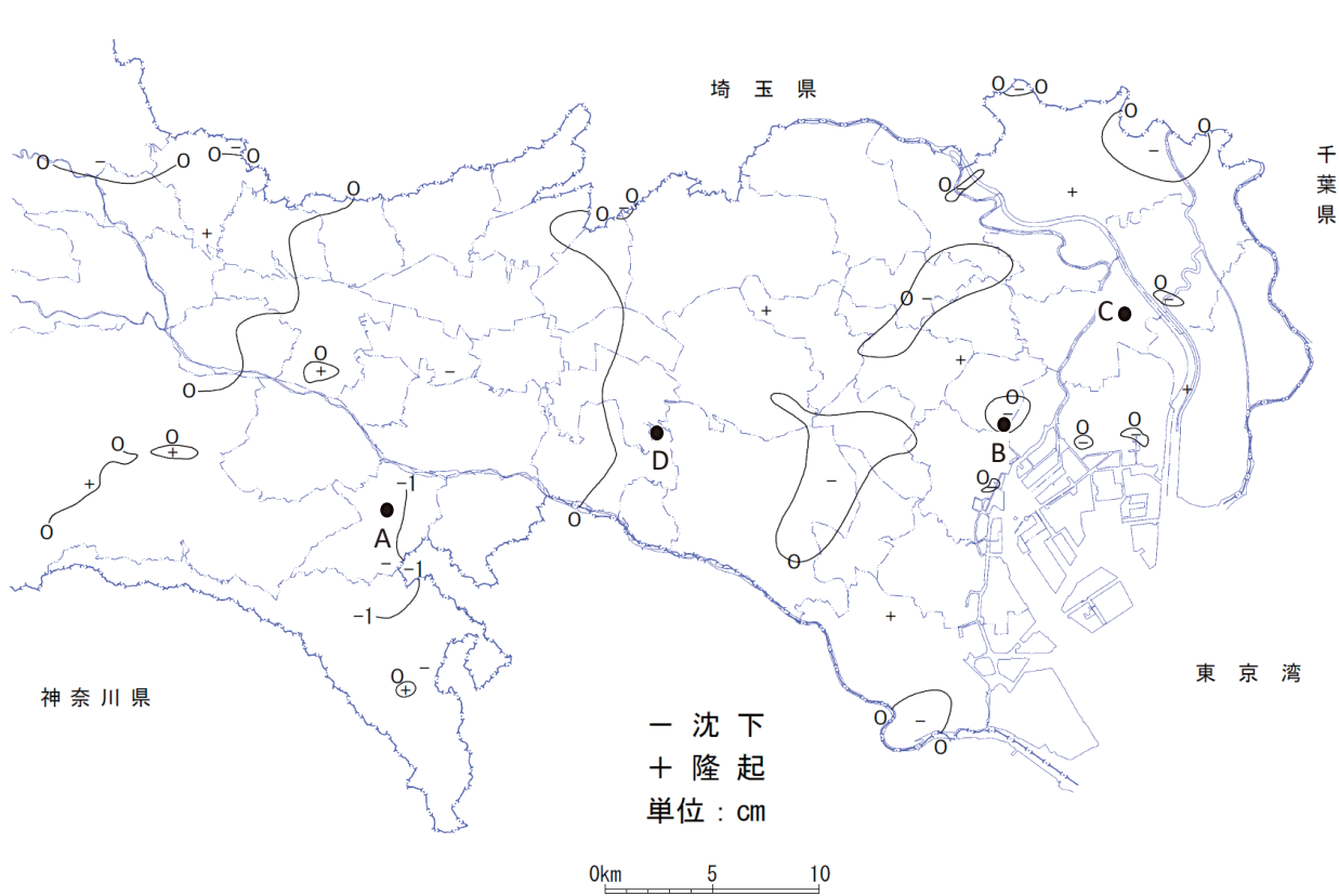
図-2 令和3年の地盤変動量図
