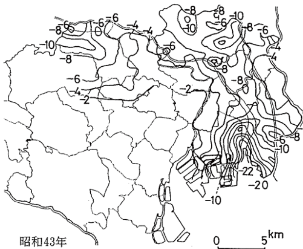
図-17 区部の地盤変動状況の変遷
