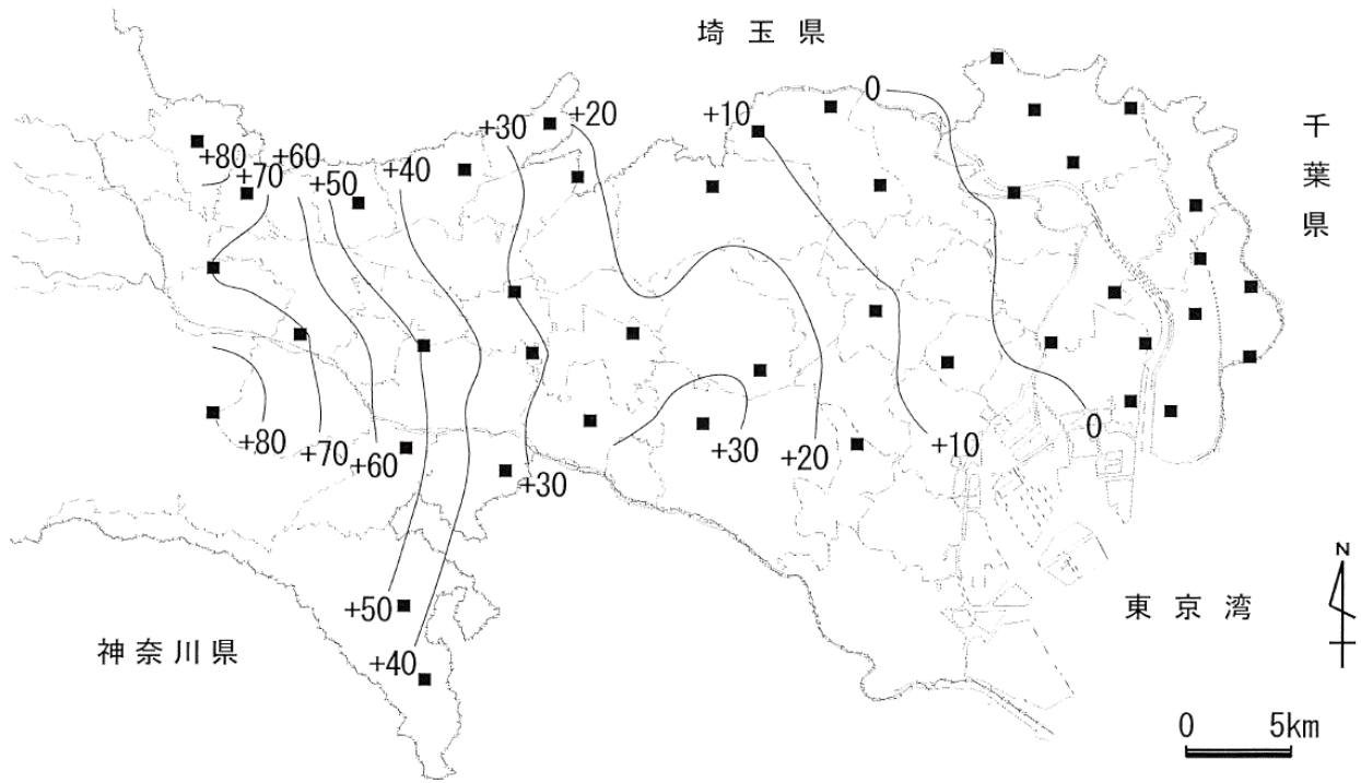
図-5 令和3年末の地下水位等高線図
