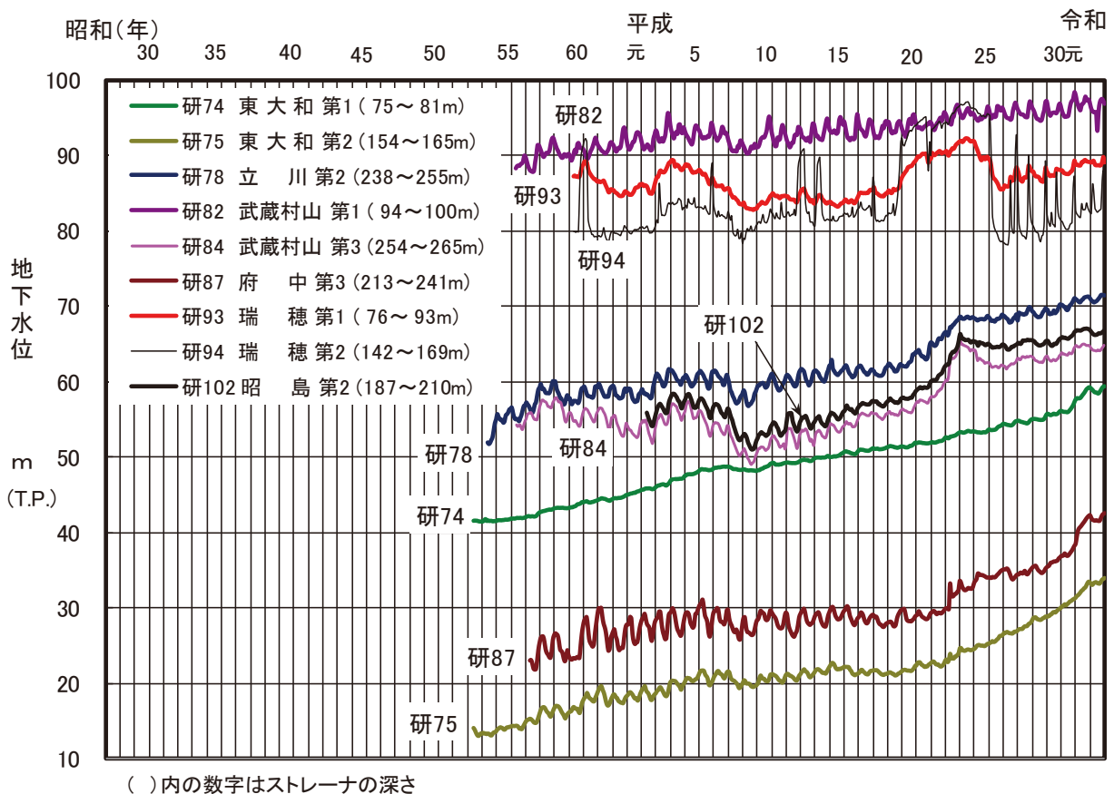
図-13 主な観測井の地下水水位変動図 (東大和市、武蔵村山市、瑞穂町、昭島市、立川市、府中市)
