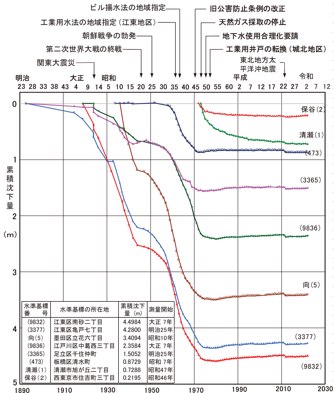
図-16 主要水準基標の累積沈下量図
