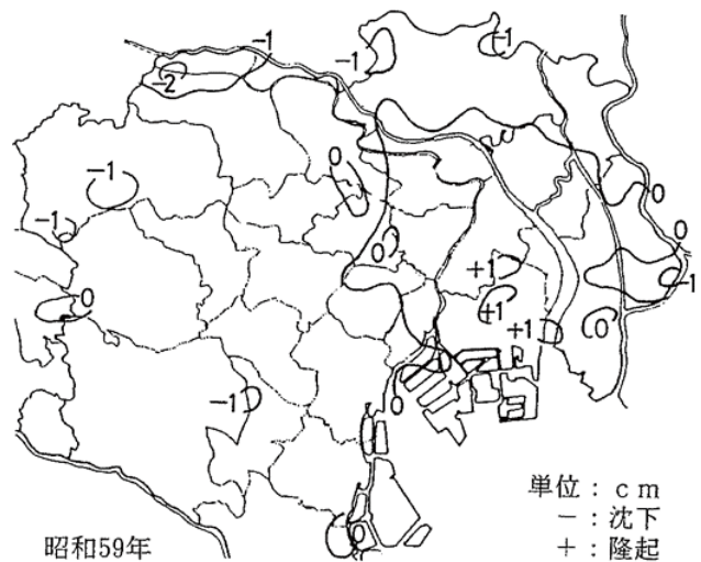
図-17 区部の地盤変動状況の変遷
