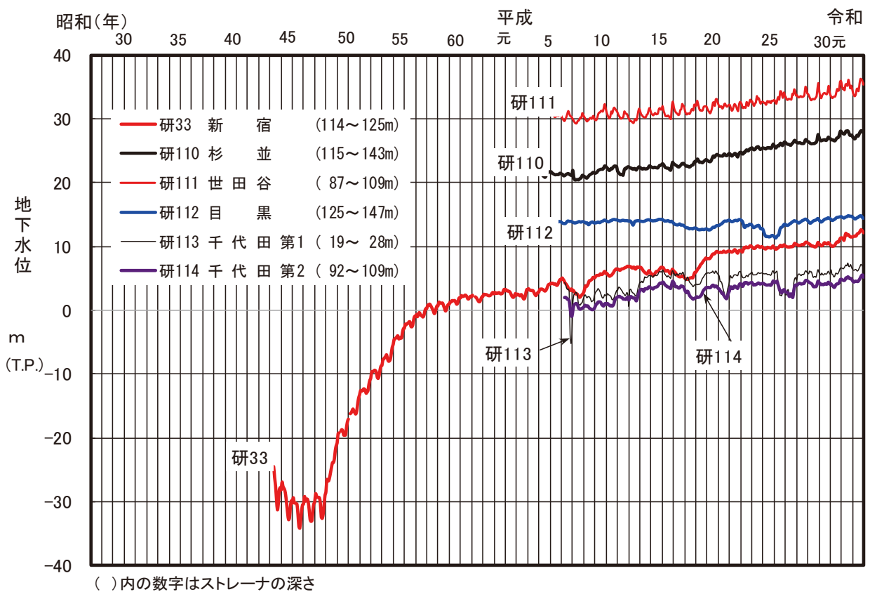
図-11 主な観測井の地下水位変動図（新宿区、杉並区、世田谷区、目黒区、千代田区）
