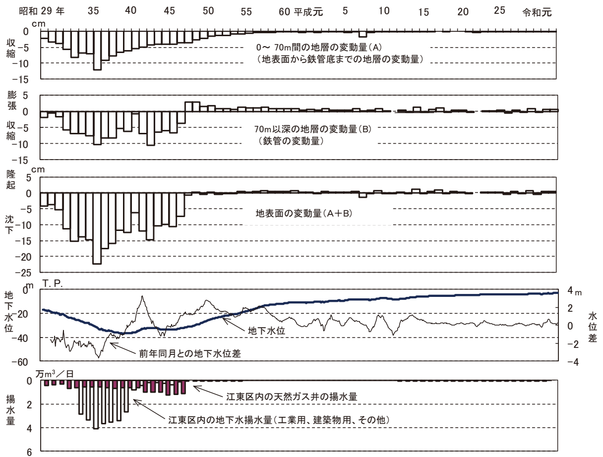
図-18 南砂町第1観測井(70m井)における地盤変動量と地下水位との関係
