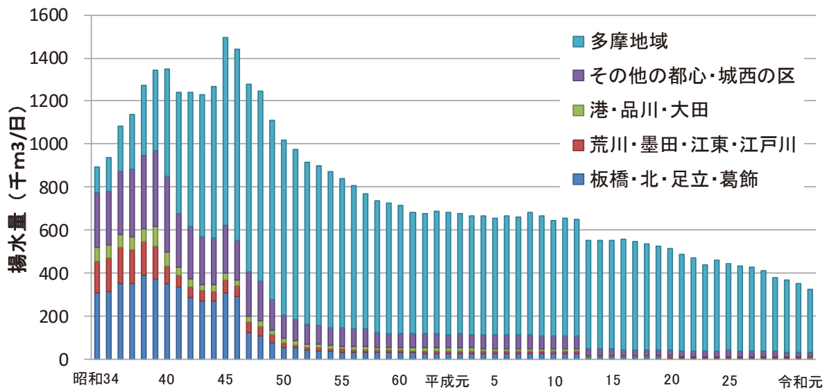
図一7 都内の地区別地下水揚水量の推移
