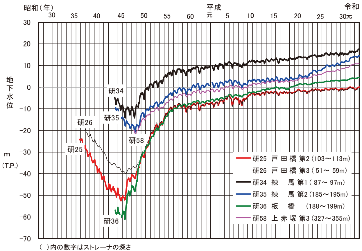
図-10 主な観測井の地下水位変動図（板橋区、練馬区）
