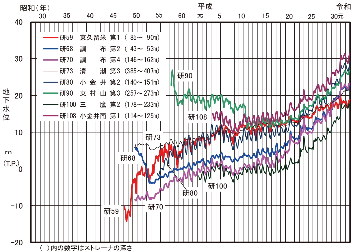
図-12 主な観測井の地下水水位変動図 (東久留米市、清瀬市、東村山市、小金井市、調布市、三鷹市)
