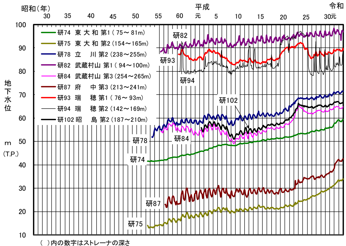
図-12 主な観測井の地下水位変動図（東大和市、武蔵村山市、瑞穂町、昭島市、立川市、府中市）
