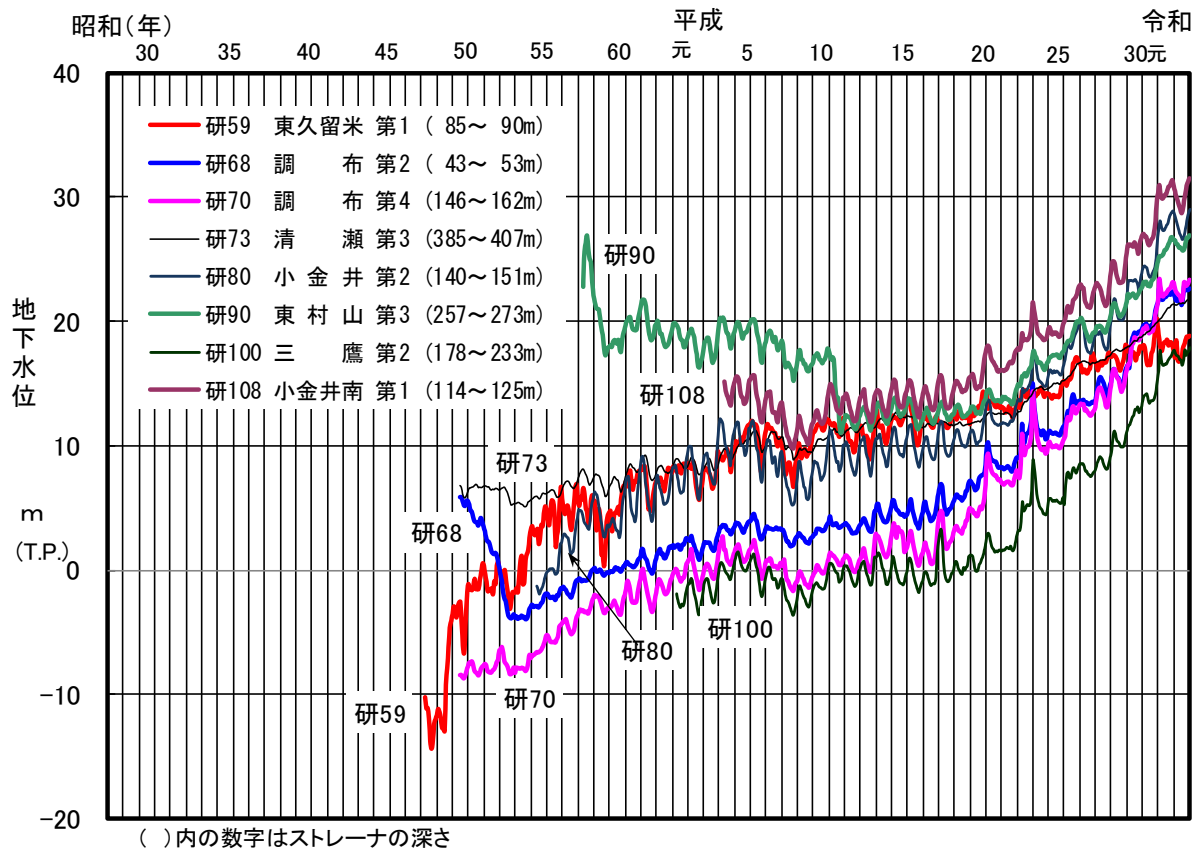
図-11 主な観測井の地下水位変動図（東久留米市、清瀬市、東村山市、小金井市、調布市、三鷹市）
