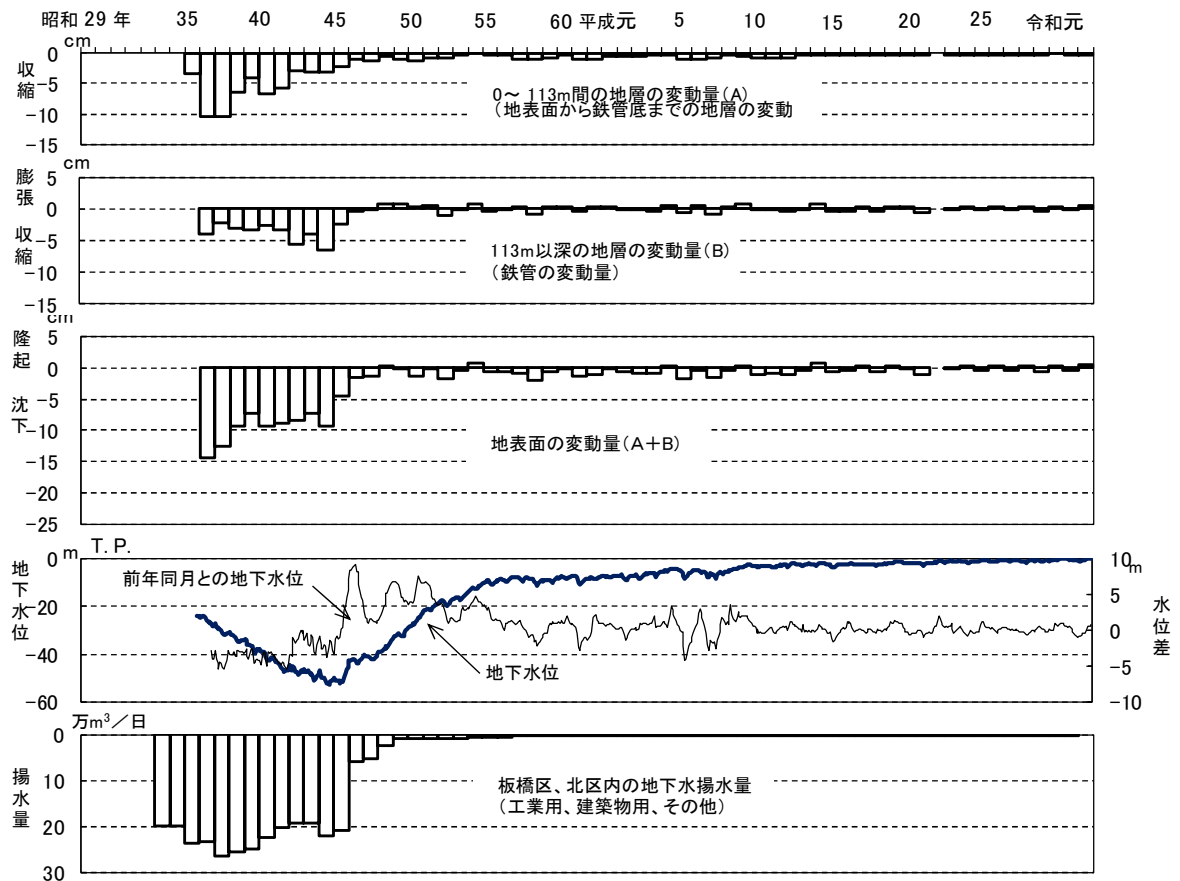
図-18 戸田橋第2観測井(113m井)における地盤変動量と地下水位との関係
