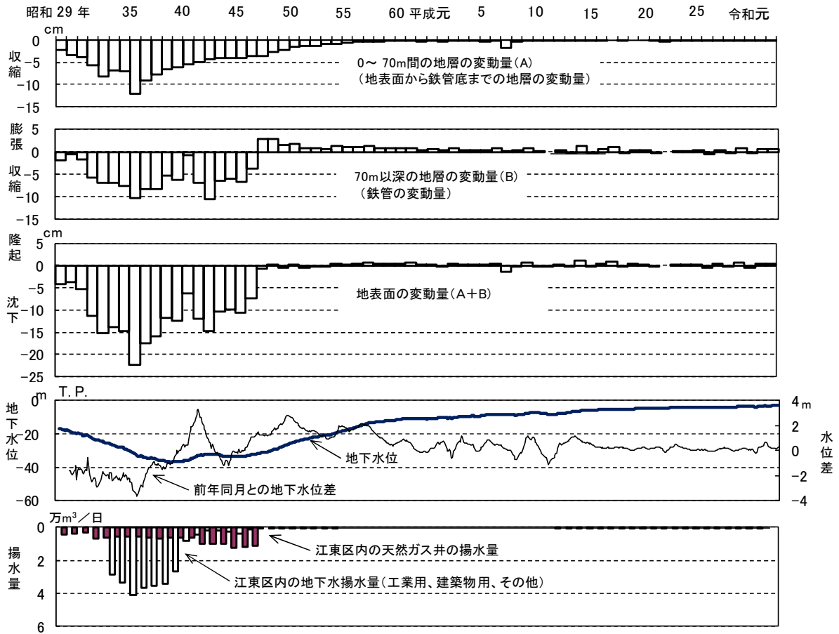
図-17 南砂町第1観測井(70m井)における地盤変動量と地下水位との関係
