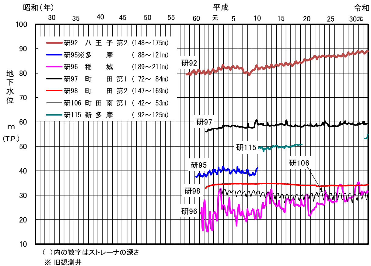
図-13 主な観測井の地下水位変動図（八王子市、多摩市、稲城市、町田市）
