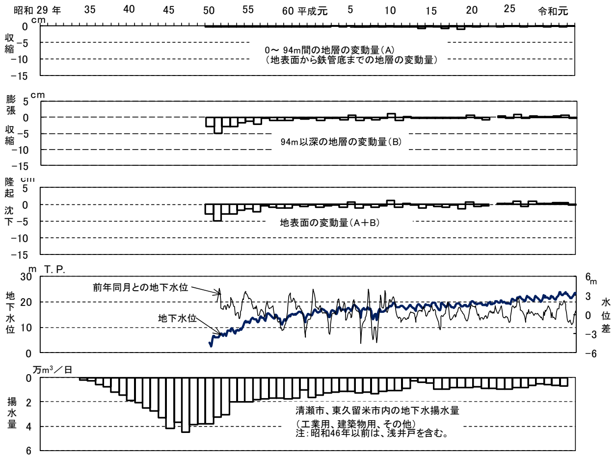
図-20 清瀬第1観測井(94m井)における地盤変動量と地下水水位との関係
