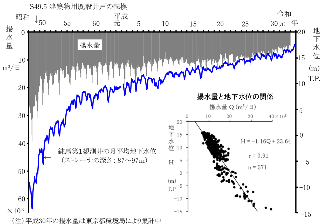
図-14 練馬区内の揚水量と地下水水位との関係
