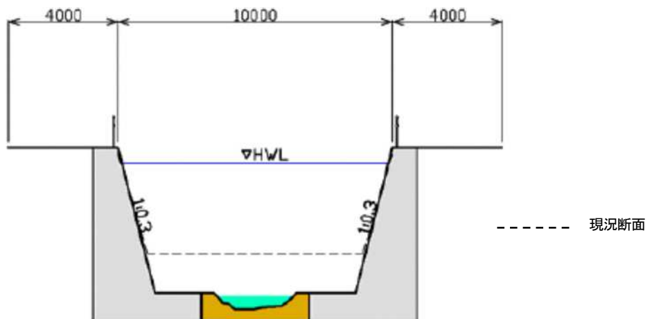
図4-1 標準断面図(神田川)
