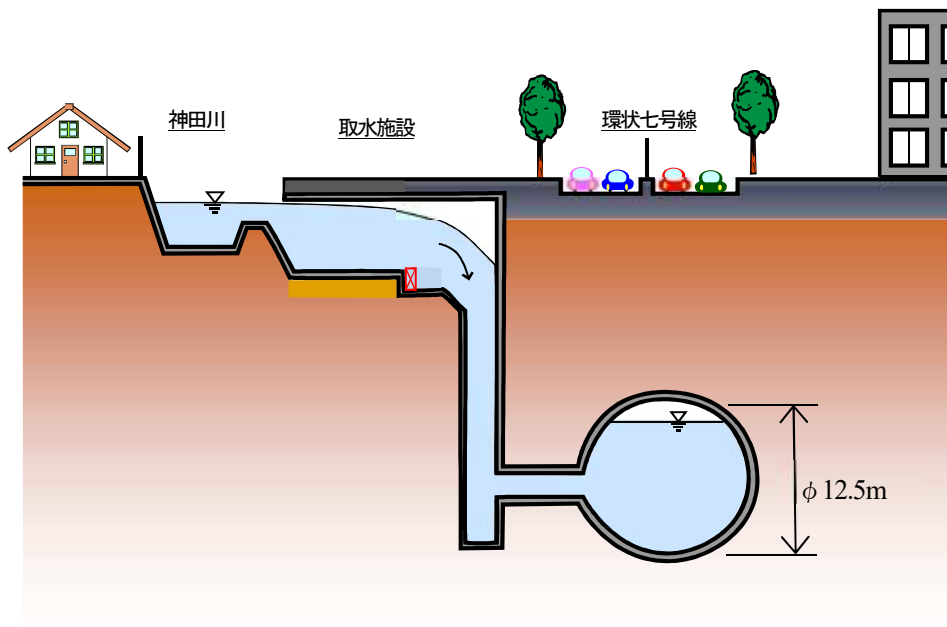
图2-3 神田川・環状七号線地下調節池概念図
