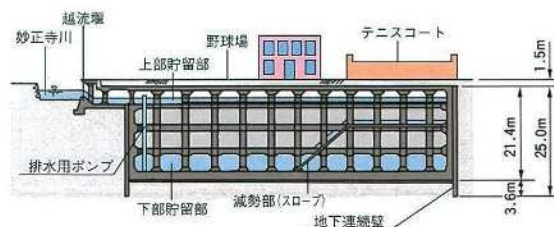
図2-10 上高田調節池 断面図
