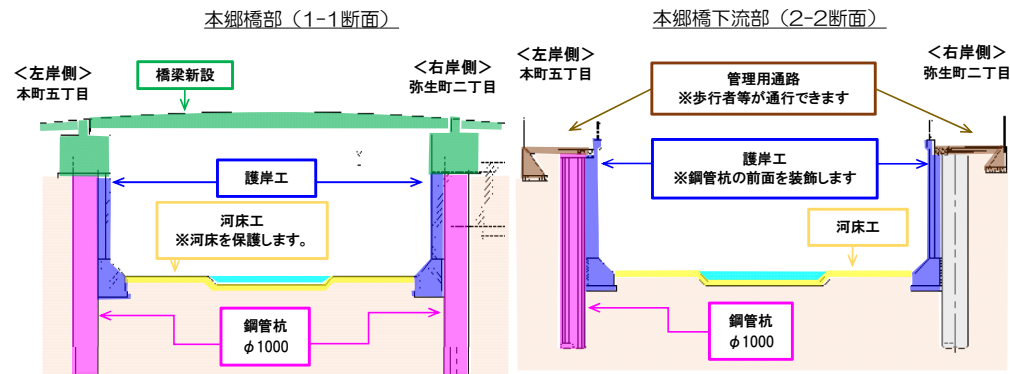
今回工事の完了断面図
