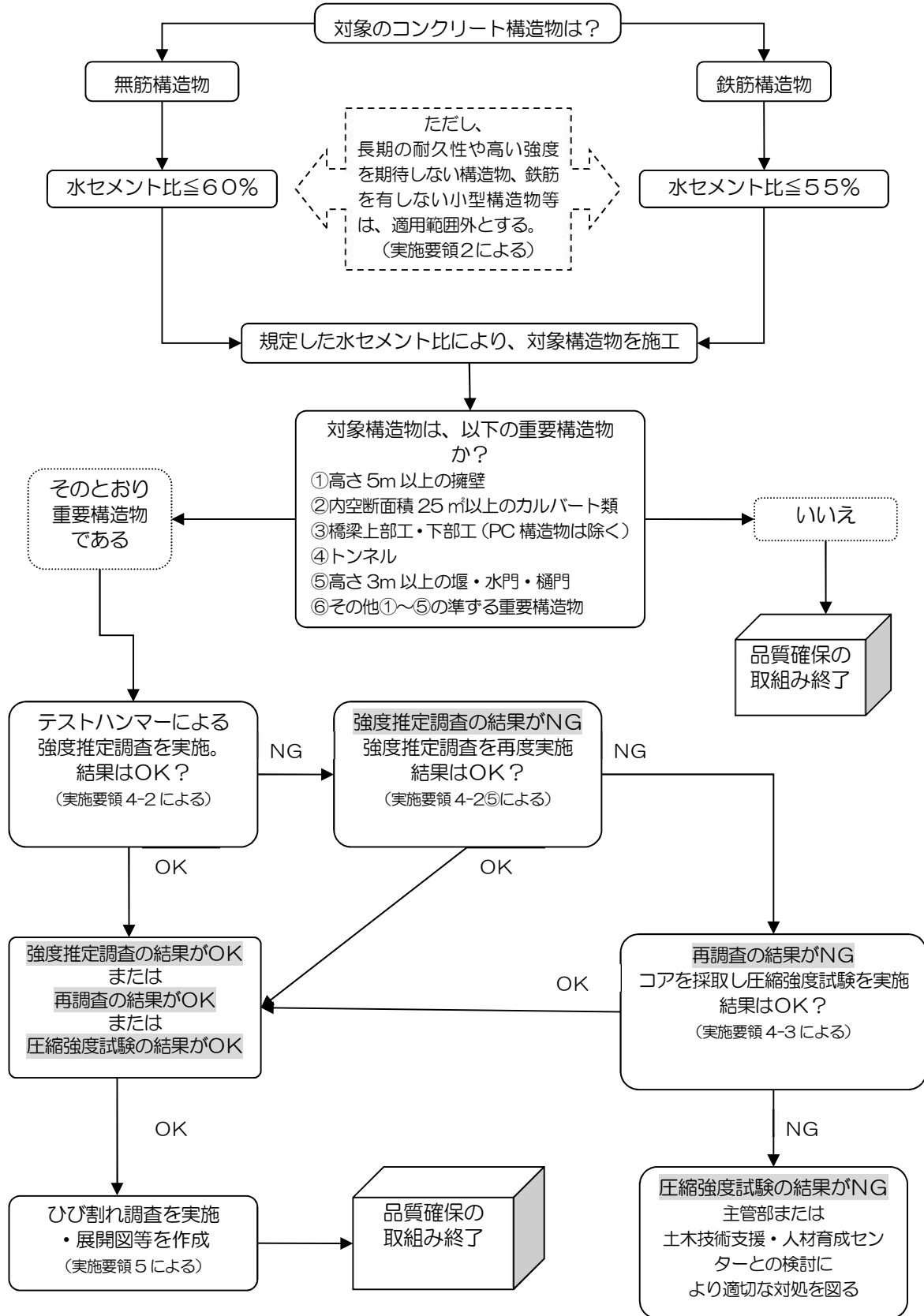
図1 「土木コンクリート構造物の品質確保」実施フロー
