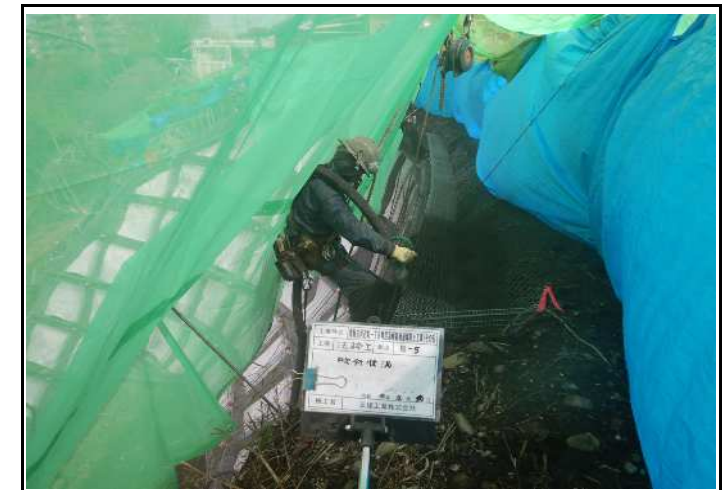
モルタル吹付時の養生状況
