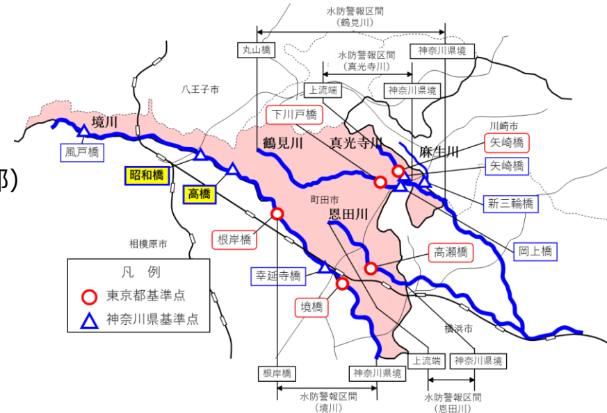
【水防警報区間と基準点位置図】
