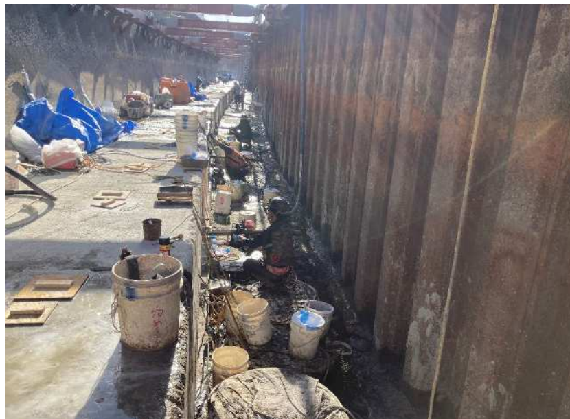
②接続鉄筋工
