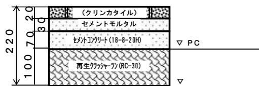
歩道 タイル舗装（例）
