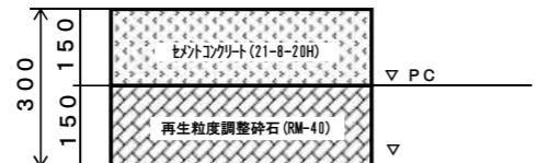
歩道 乗入れ舗装（区分：A、B、C） （セメコン・30型）
