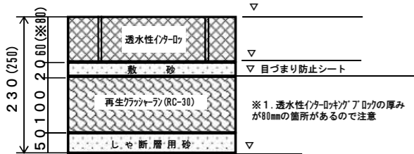
歩道 インターロッキングブロック舗装（透水性）
