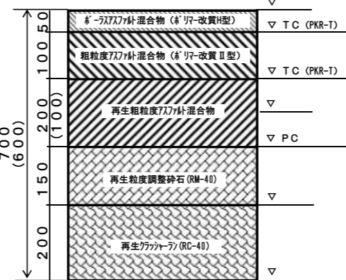
車道 アスファルトコンクリート舗装 （低騒音・70（60）型）
