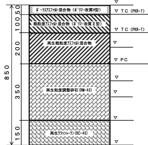
車道 アスファルトコンクリート舗装 （低騒音・70（60）型）
