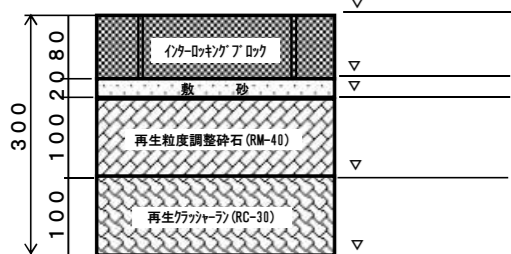
歩道 乗入れインターロッキングブロック舗装 （区分：A、B、C）（非透水性・30型）
