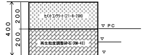
歩道 乗入れ舗装（区分：D） （セメコン・40型）
