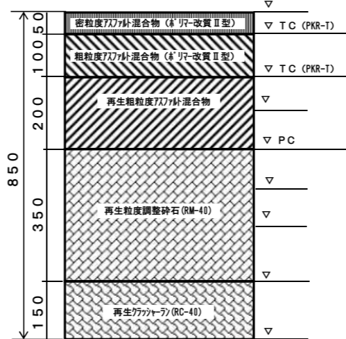
車道 アスファルトコンクリート舗装 （改質Ⅱ型・70（60）型）
