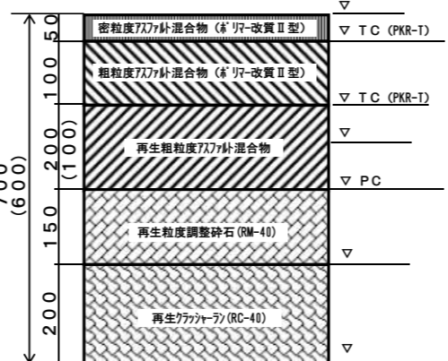
車道 アスファルトコンクリート舗装 （改質Ⅱ型・70（60）型）
