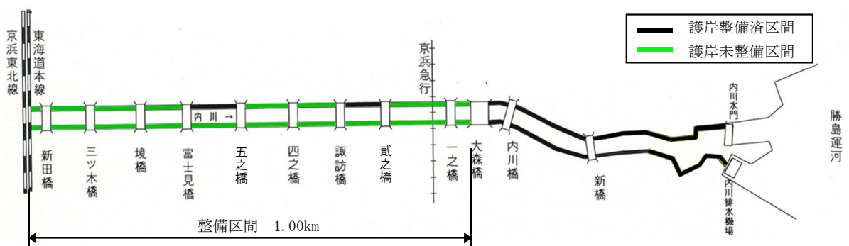
図 4-3 整備箇所図
