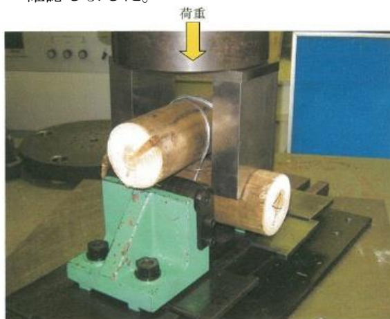
写真 - 5 ①鉄線(二重縄掛け)固定
