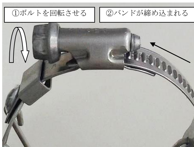
写真 - 2 ボルトを回転させて締め込む構造
