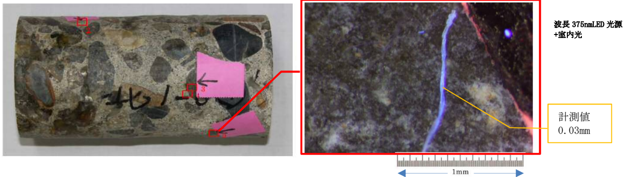
写真-2 ひび割れ幅計測写真
