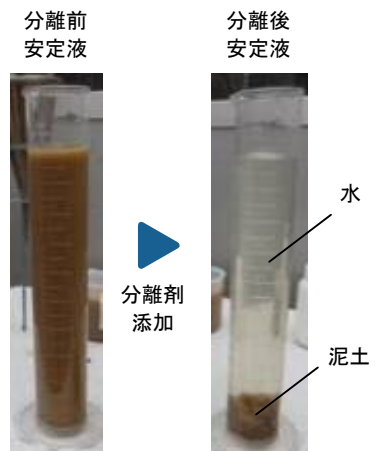
サプリ安定液の分離 (水と泥土に分離)
