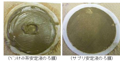
写真-1 各安定液で形成された泥膜
