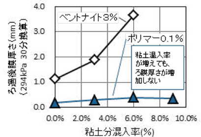
図-4 安定液粘土混入率と泥膜厚
