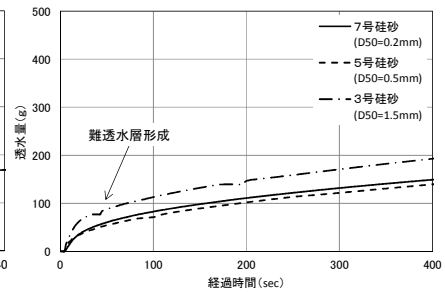
図-3 透水量経時変化 (サプリ安定液)
