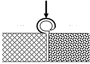
図-1 サスエッジの載荷試験法
