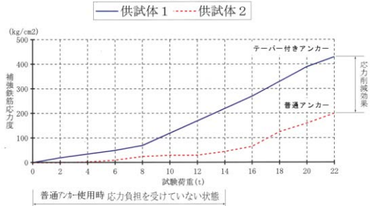
応力度比較
